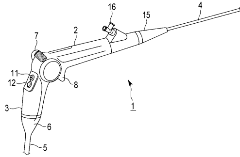
【 図 4 B 】
