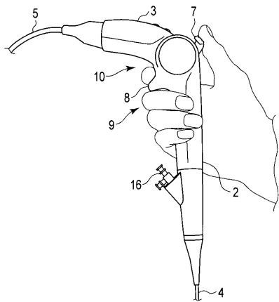
【 図 9 B 】
